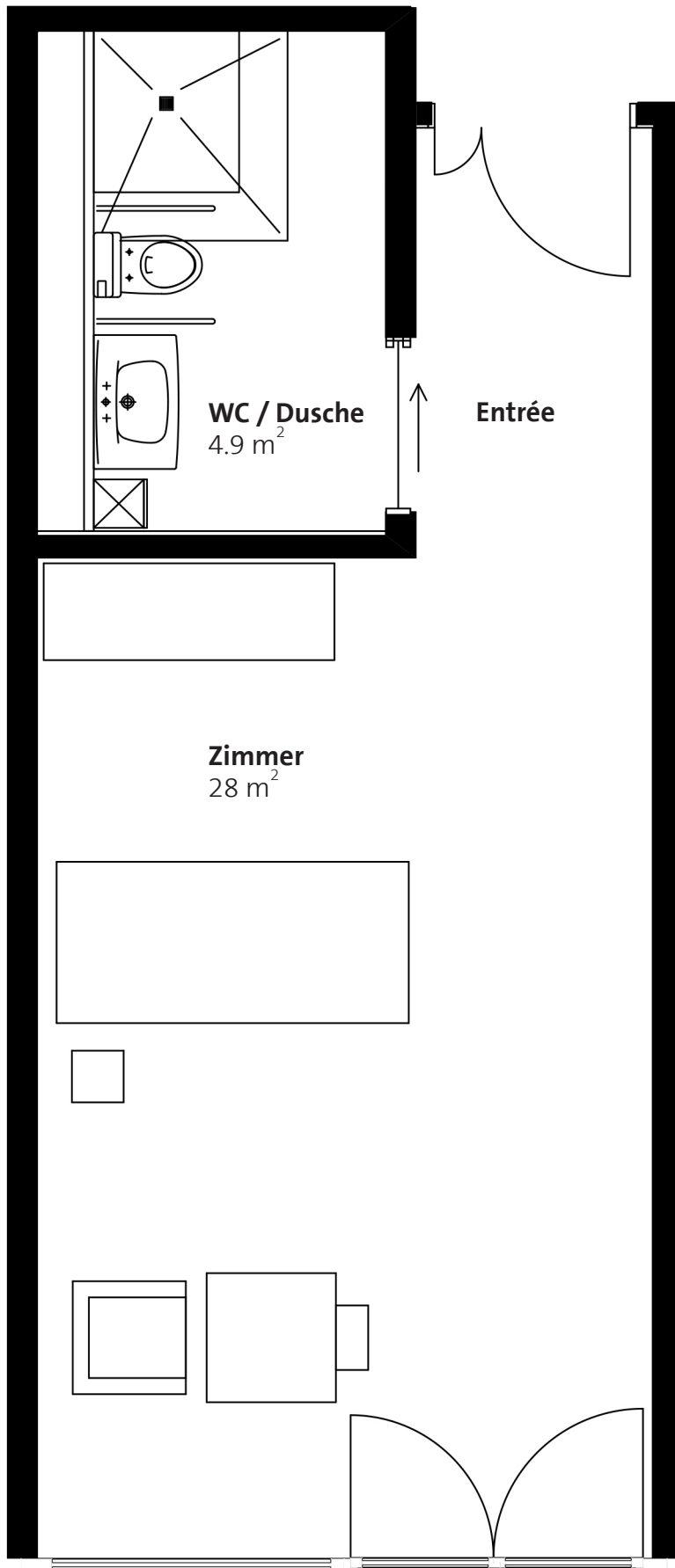
Pflegezimmer mit 33 m 2 | Mst: 1:100
